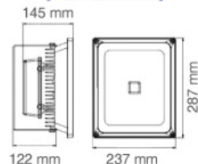
[FZL-FL60-00-60]
